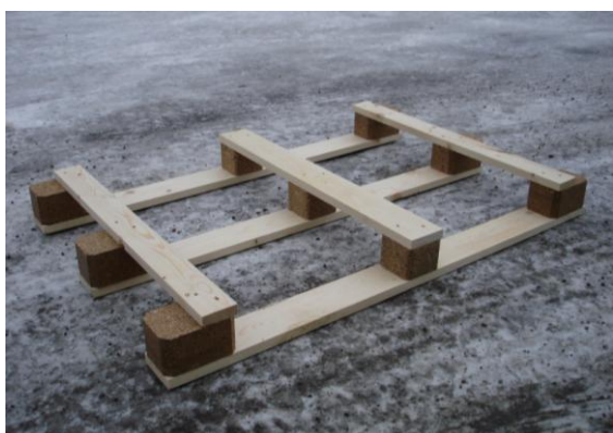
Pall A för 4-vägs hantering
